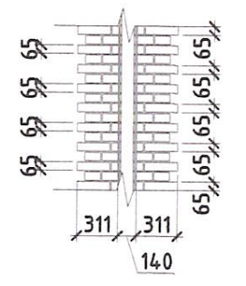
Фрагмент "12" Узорная полоса выступает на - 25 мм (существующая)
