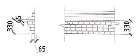
Фрагмент "18" Карниз из кирпича h=330 мм (существующий)
