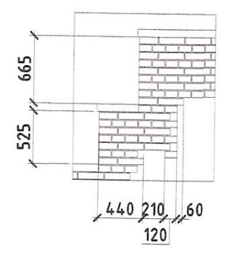
Фрагмент "15" Узор из кирпичной кладки (существующий)
