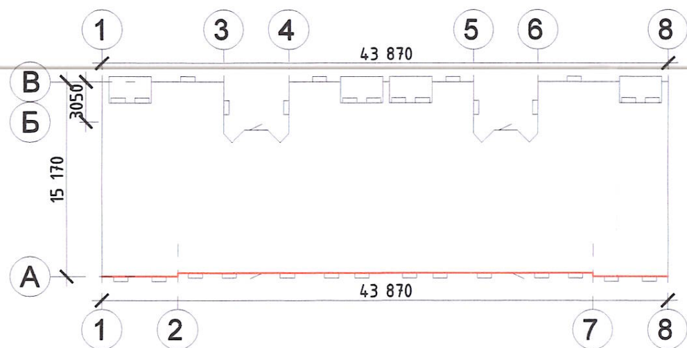
Схема здания
