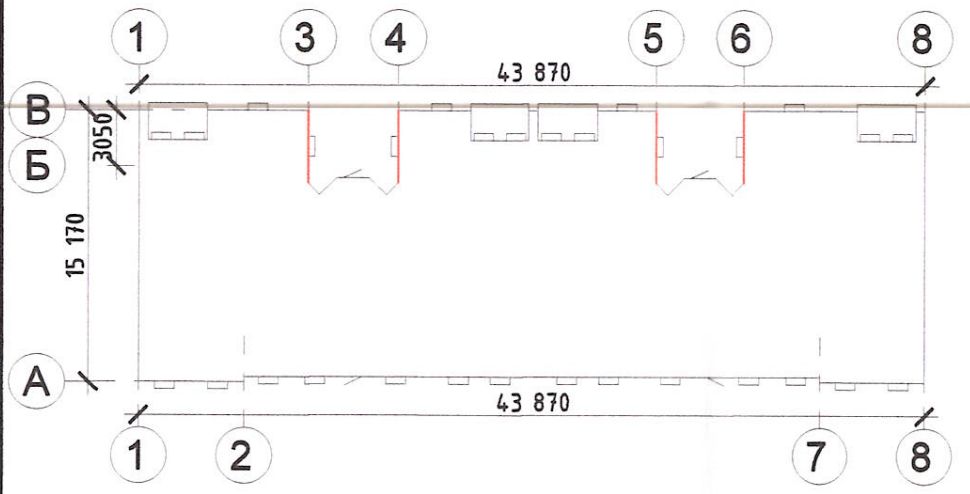
Схема здания
