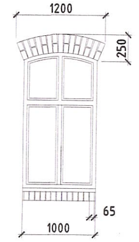
Фрагмент "16" Имитация кладки лучковых перемычек и подоконных элементов (повторяющая сущ-ю кладку) выполнено декоративной штукатуркой по трафарету
