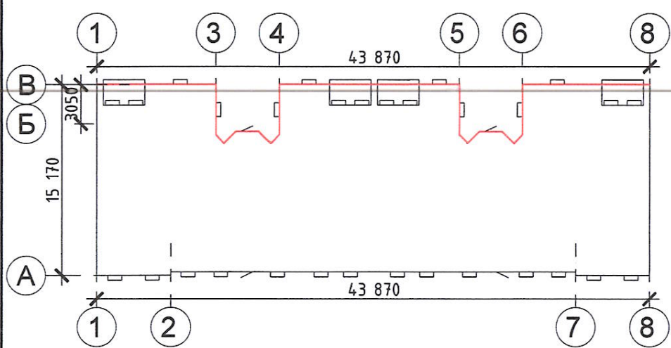
Схема здания
