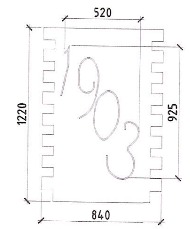
Фрагмент "20" Прорезной декор, шириной и глубиной 30мм, плоскость вокруг декора отделать гладкой штукатуркой (существующий)
