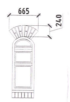
Фрагмент "19" Имитация кладки лучковых перемычек (повторяющая сущ-ю кладку) выполнено декоративной штукатуркой по трафарету
