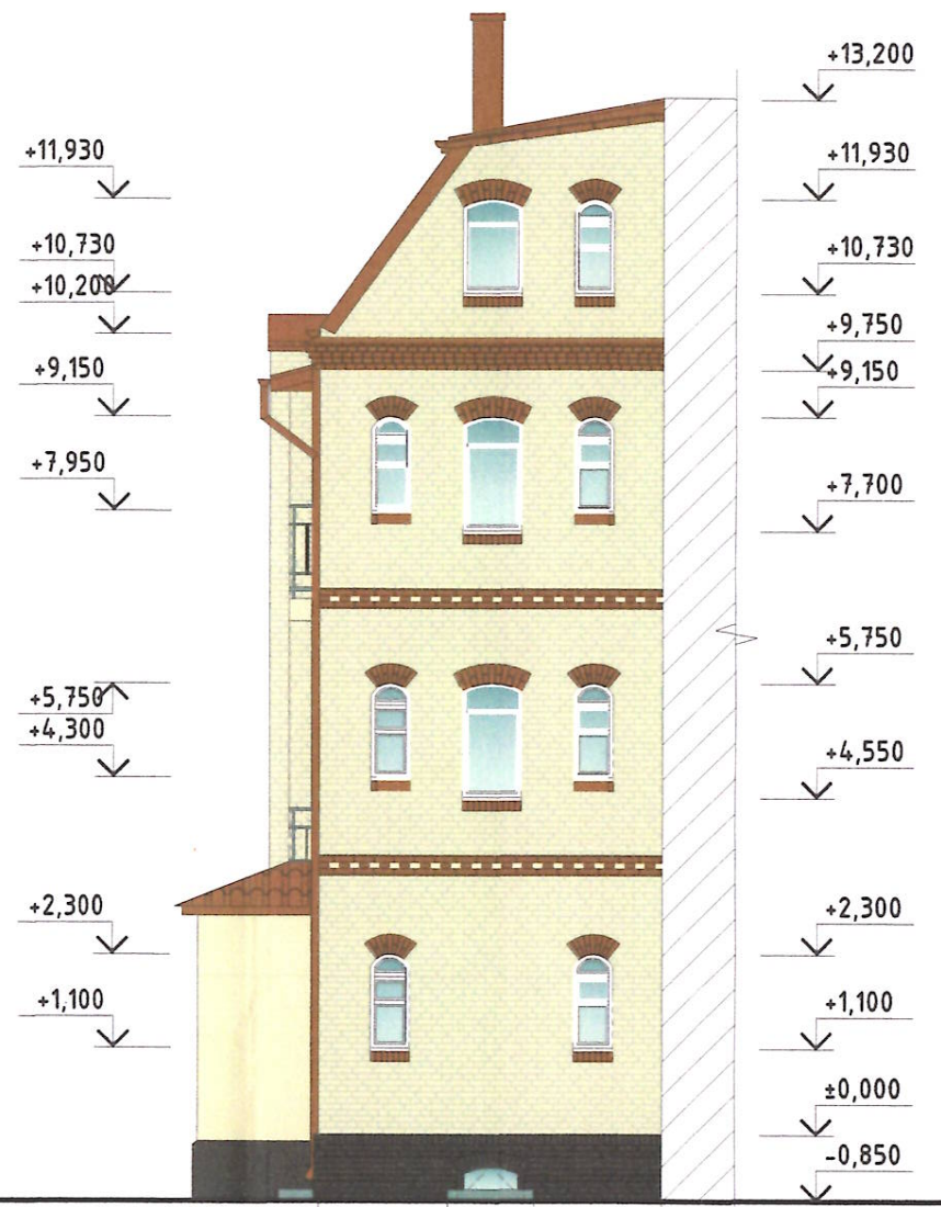
Цветовое решение фасада по оси 6 М 1:100
