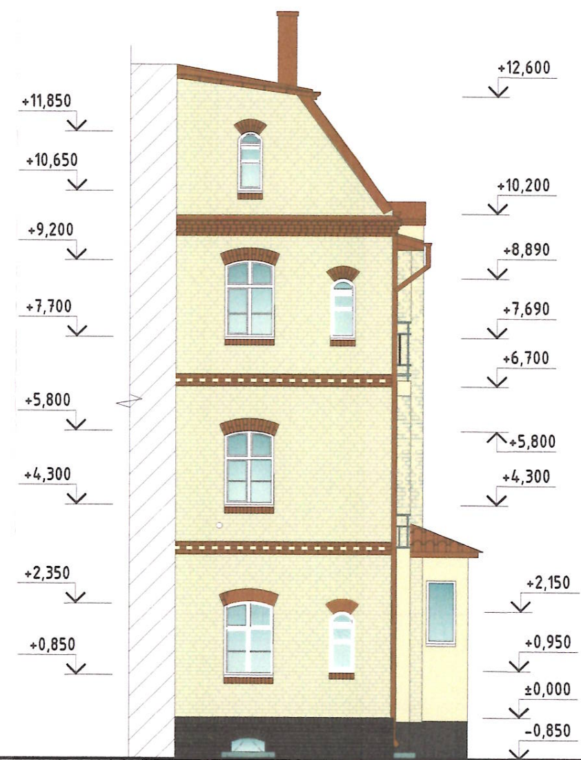
Цветовое решение фасада по оси 5 М 1:100
