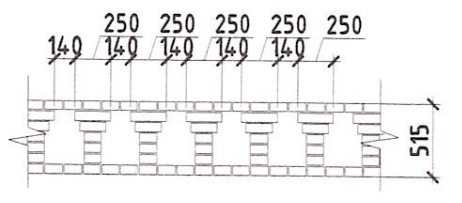
Фрагмент "13" Карниз кирпичный "Сухарики" (существующий)
