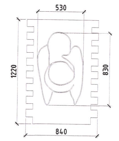
Фрагмент "21" Прорезной декор, шириной и глубиной 30мм, плоскость вокруг декора отделать гладкой штукатуркой (существующий)
