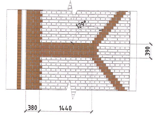
Фрагмент "14" Узор из кирпичной кладки (существующий)
