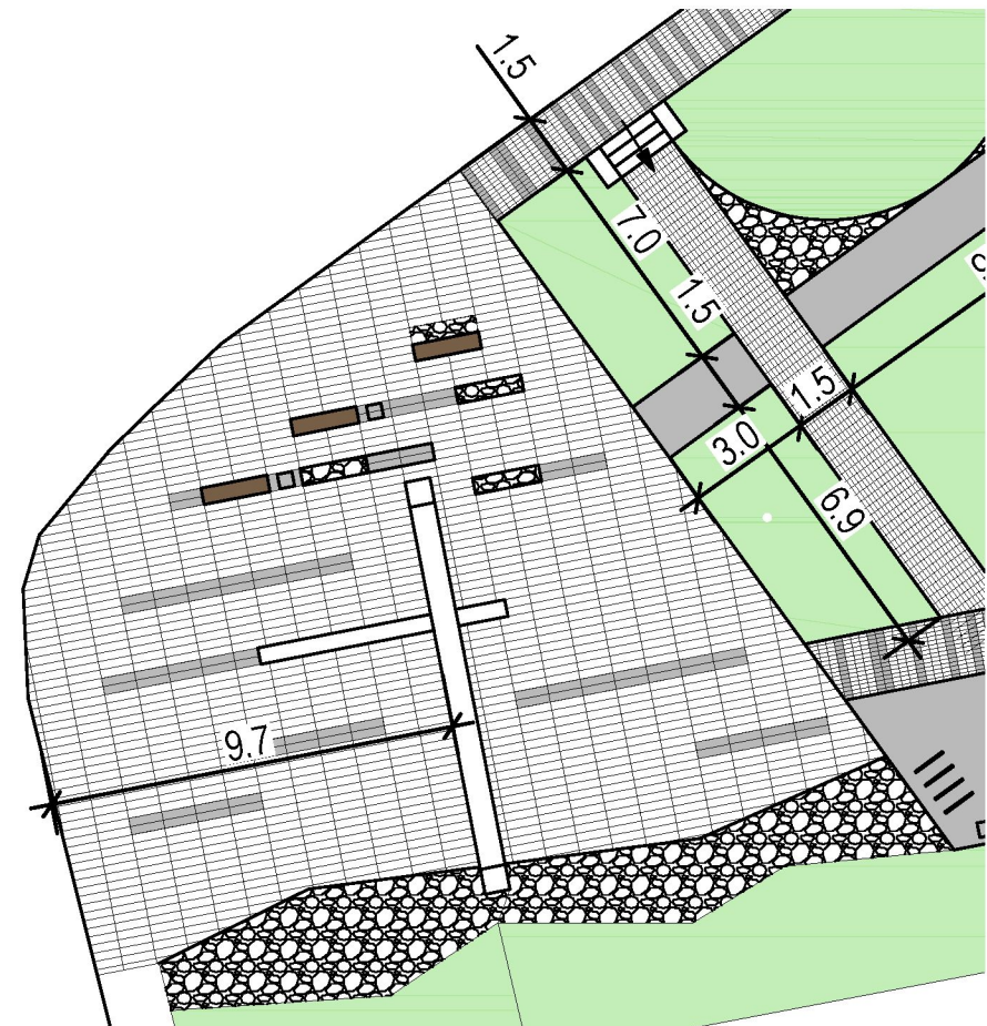
Фрагмент 2. Площадка отдыха М 1:200
