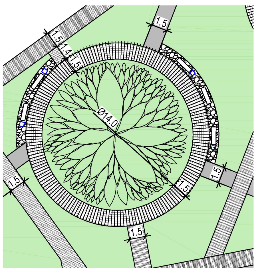
Фрагмент 3. Входная группа М 1:200
