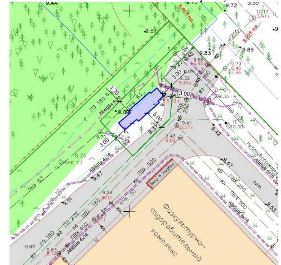
схема размещения культового здания в границах земельного участка
