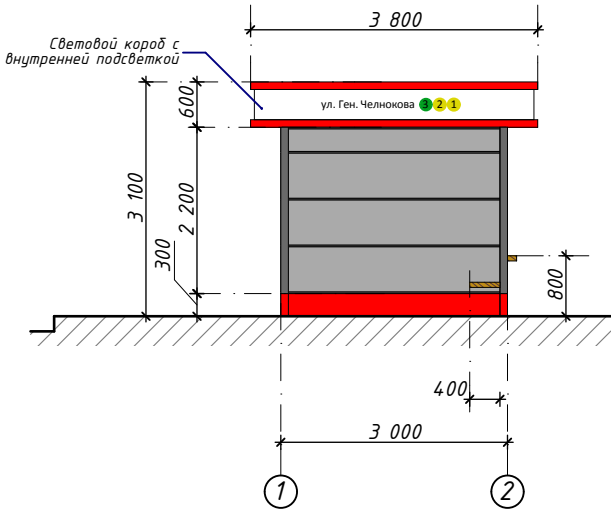
Фасад в осях 1-2
