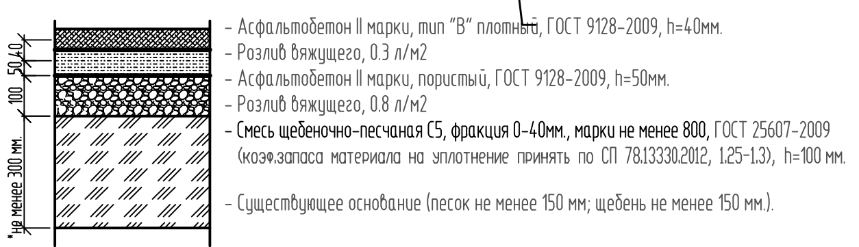
Тип 3 (Конструкция дорожной одежды для устройства проезжей части из асфальтобетонного покрытия, толщиной 90 мм.)
