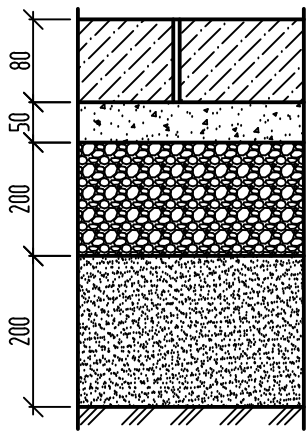
Тип 1. (Конструкция дорожной одежды для устройства дворового проезда из бетонной плитки, толщиной 80 мм.)
