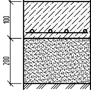
Тип 9. (Конструкция дорожной одежды для устройства тротуара из бетона, толщиной 100 мм.)
