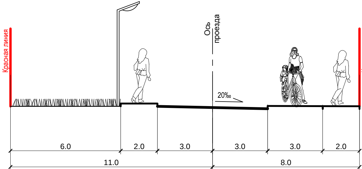
Поперечный профиль 1-1
